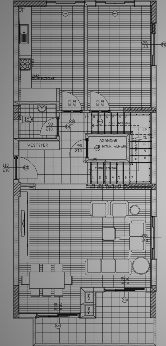
ZEMİN KAT PLANI
