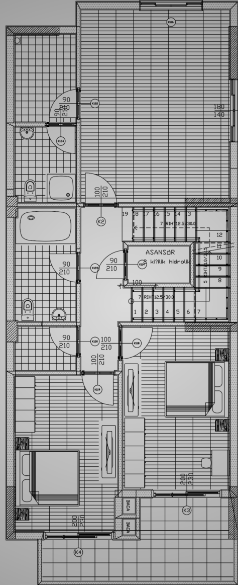
BİRİNCİ KAT PLANI
